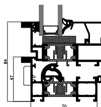
vue en coupe : fenêtre ouvrable
